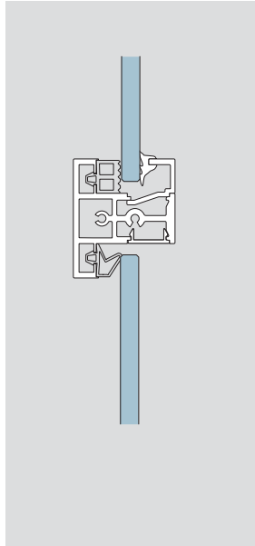
Rung profil
