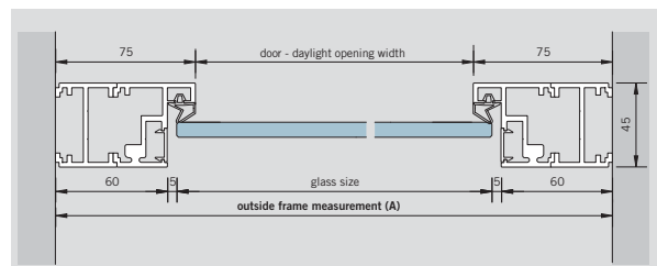
plan / door Type B
